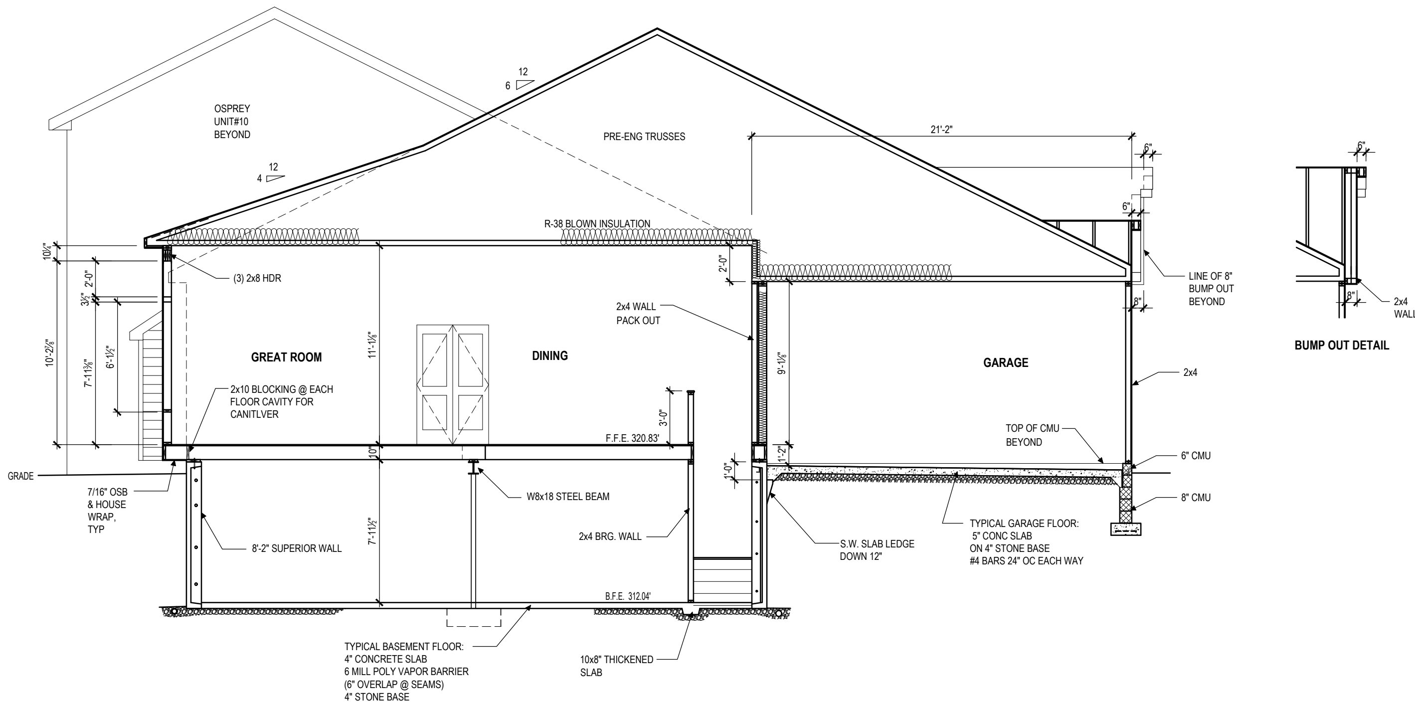
B A206 HUTTON - SECTION 'B' SCALE: 3/16"=1'-0"
