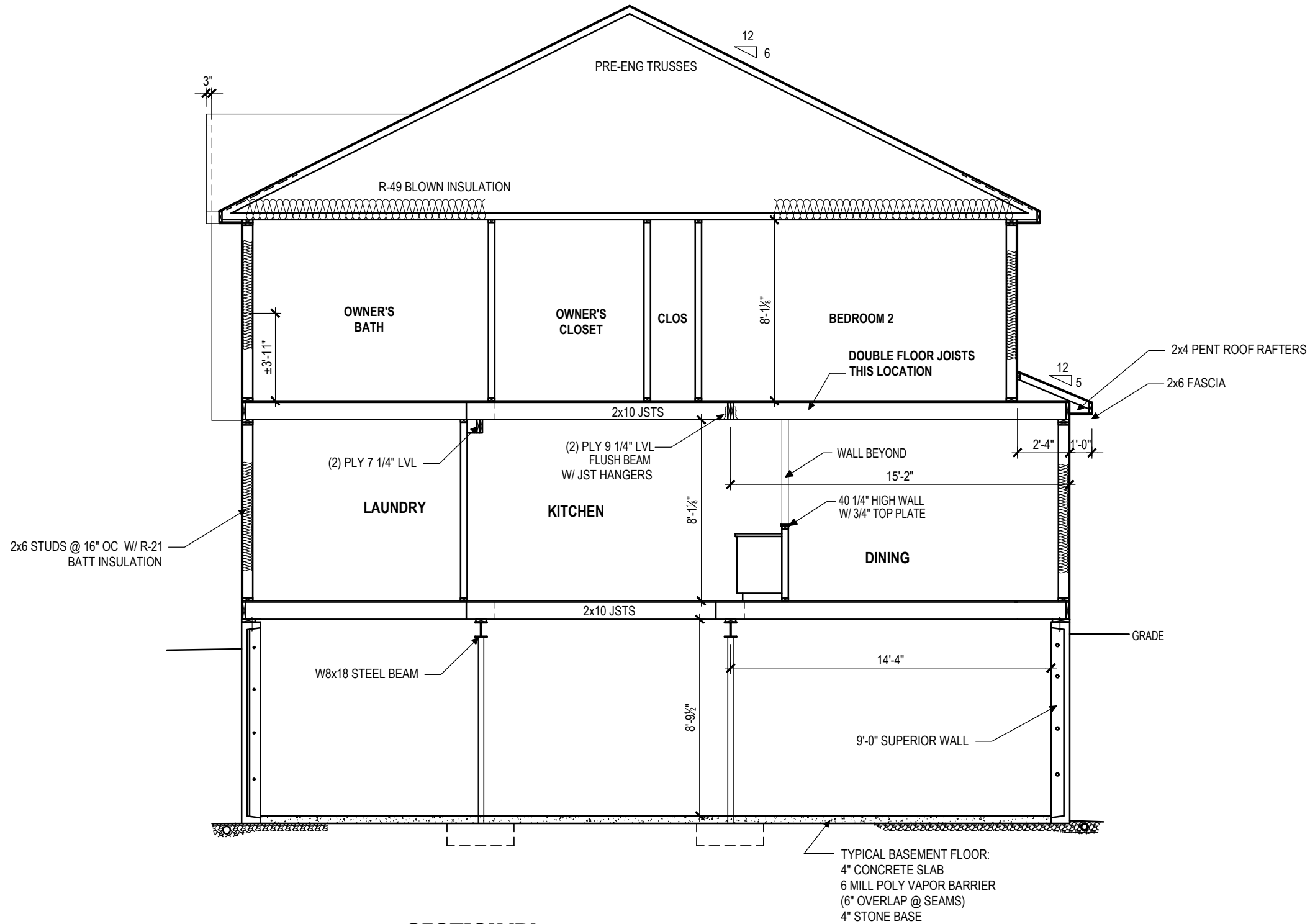
B A207 SECTION 'B' SCALE: 3/16"=1'-0"
