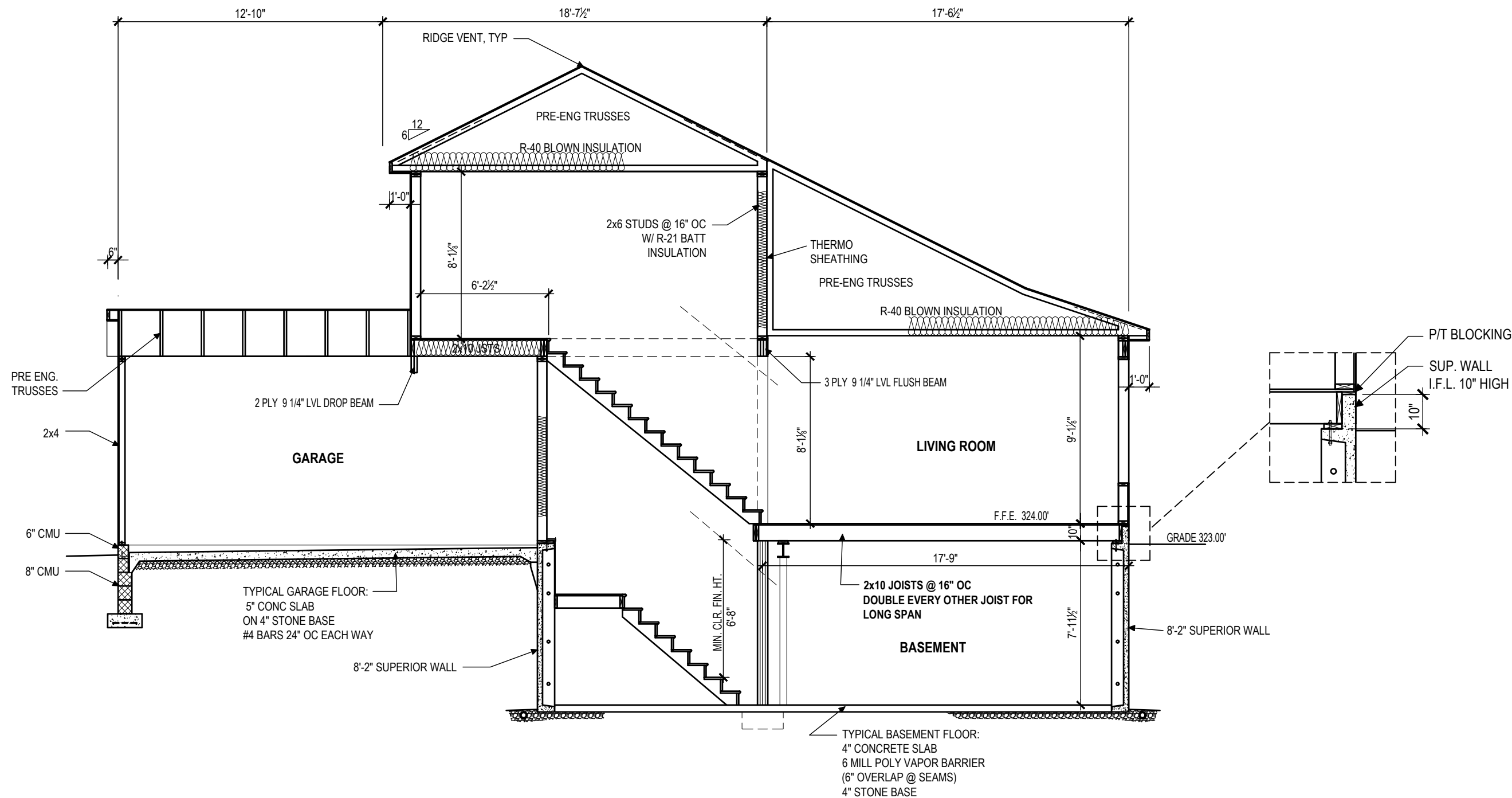
B A406 SECTION 'B' SCALE: 3/16"=1'-0"
