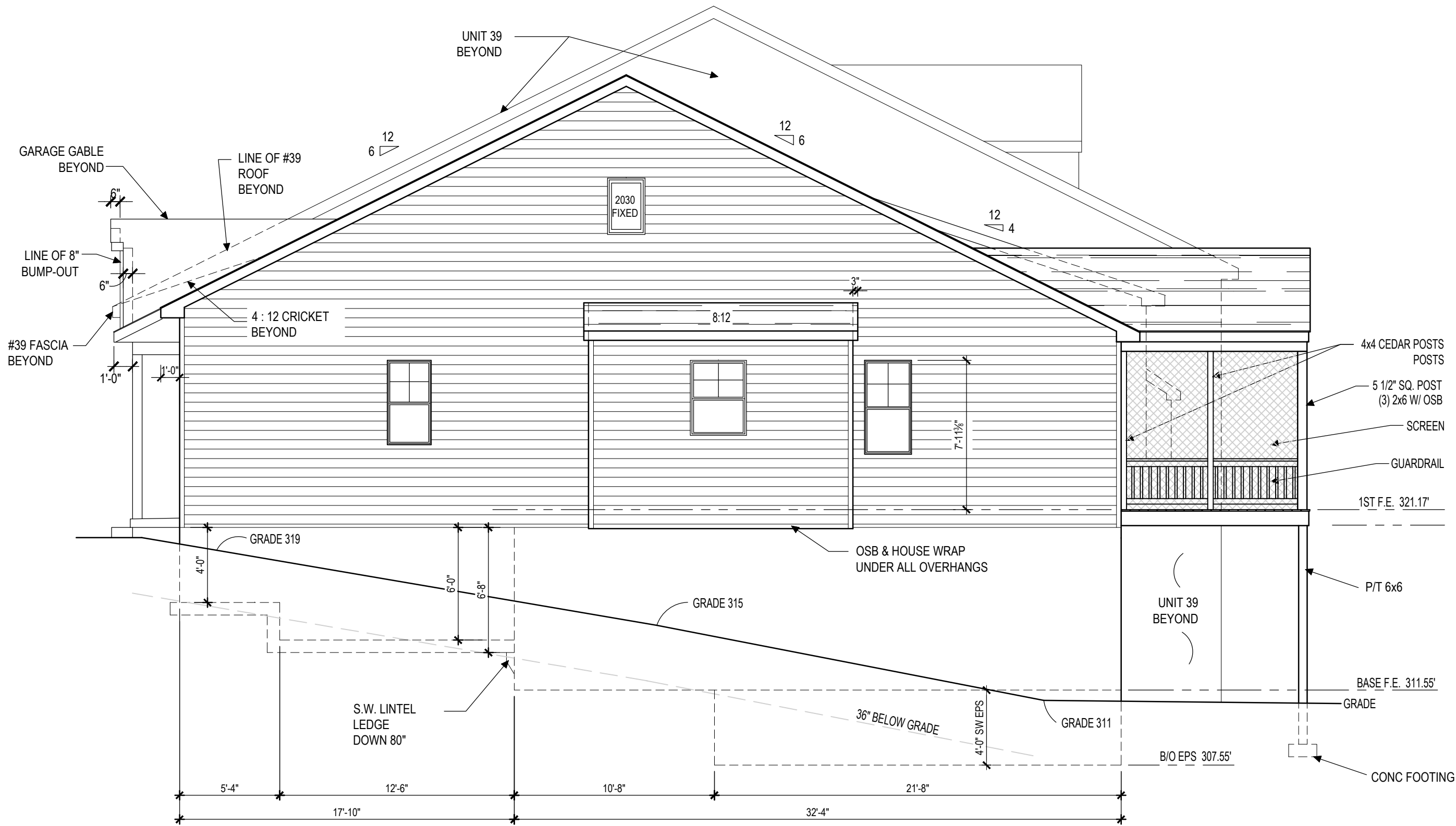
1 A404 SIDE ELEVATION SCALE: 3/16"=1'-0"
