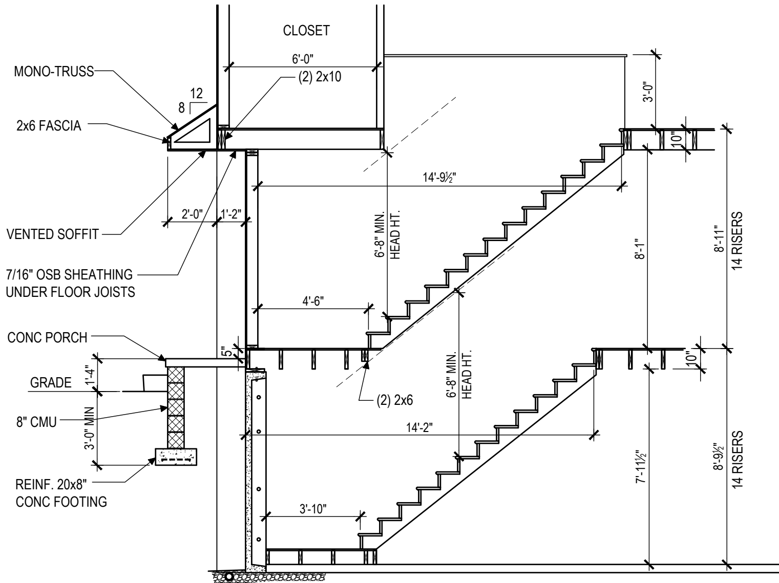
1 A507 SIDE PORCH & STAIR SECTION SCALE: 1/4"=1'-0"
