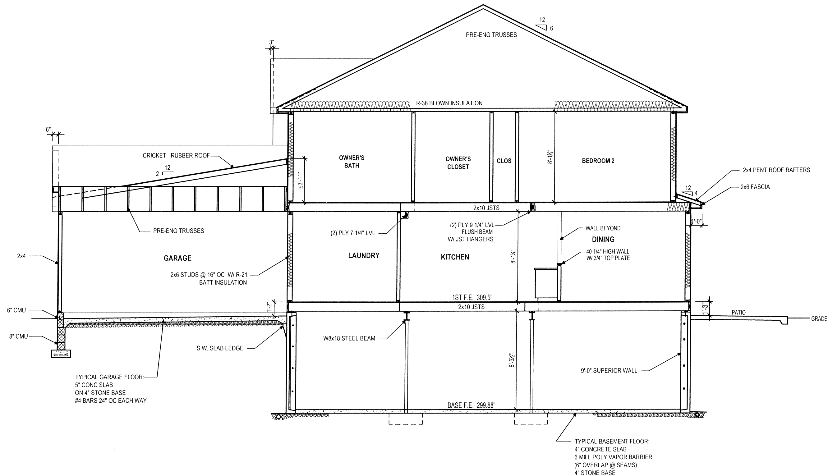
DAWN - SECTION SCALE: 3/16"=1'-0"
