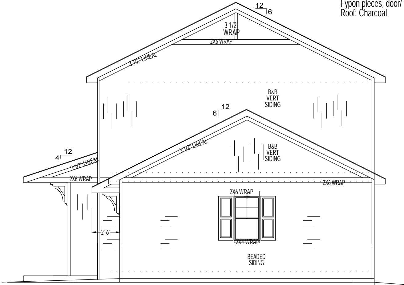
RIGHT ELEVATION
