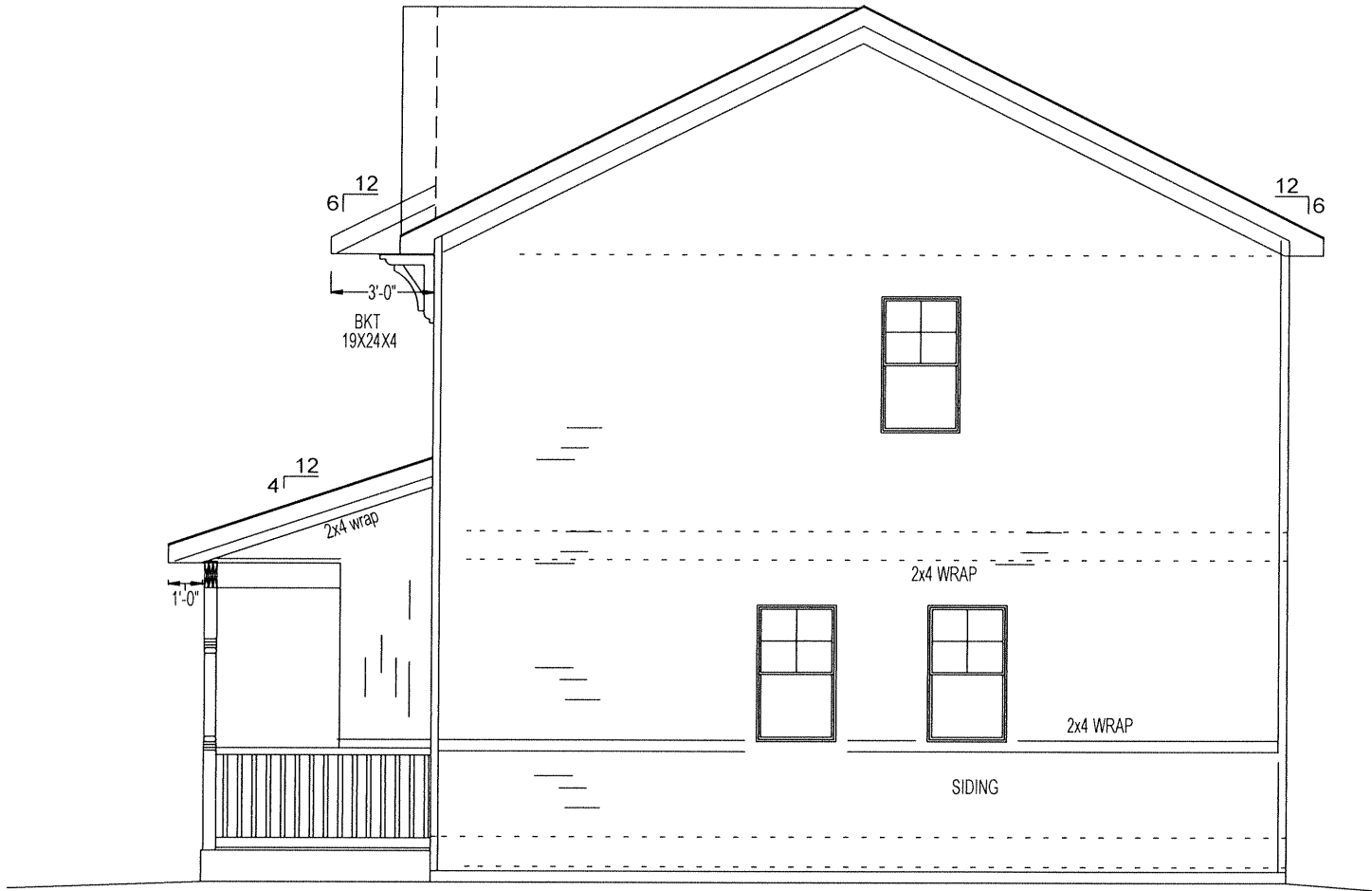
RIGHT ELEVATION
