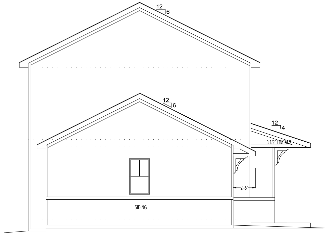
RIGHT ELEVATION
